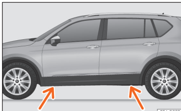
Afb. 37 Steunpunten voor de krik.
