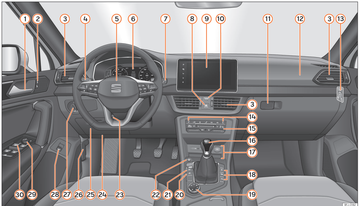
Afb. 53 Bestuurdersruimte.
