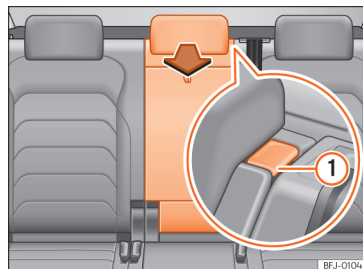
Afb. 130 Rugleuning achterin: luik voor lange ladingen openen.
