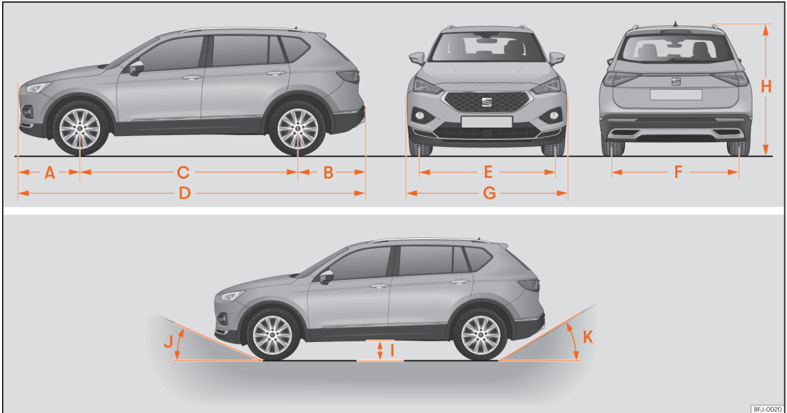
Afb. 259 Afmetingen
