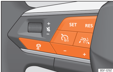
Afb. 194 Linkerzijde van het multifunctiestuurwiel: toetsen voor bediening van Travel Assist.
