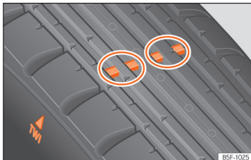
Afb. 254 Bandenprofiel: slijtagemerkttekens.
